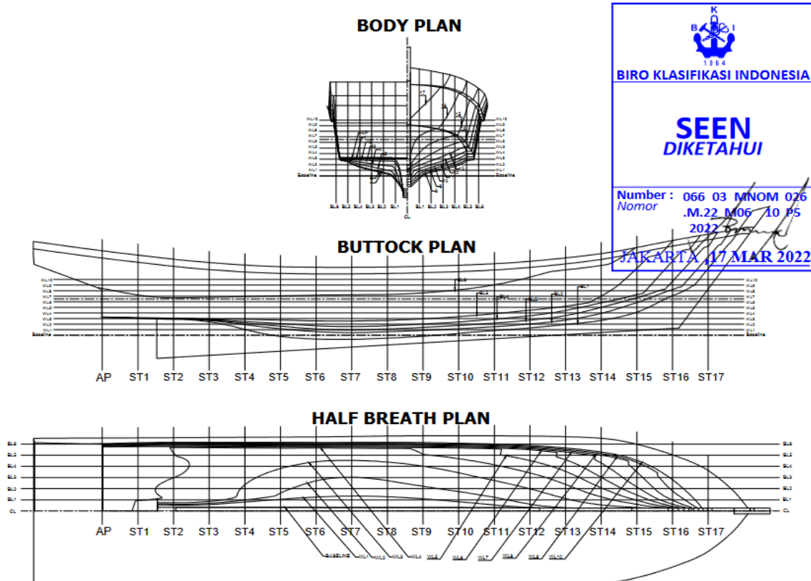
Gambar 1 : Lines plane model kapal yang sudah di setuju BKI
