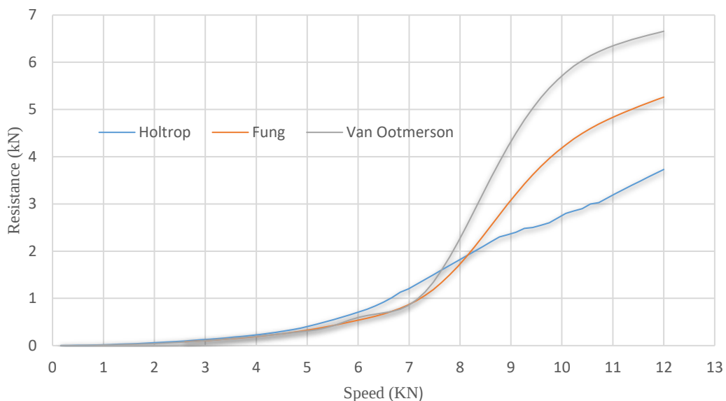
Gambar 3: Hambatan Vs Kecepatan kapal 5GT
