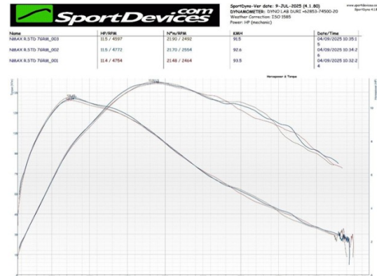
Gambar 1. Grafik Rata-rata Torsi dan Daya 7g
