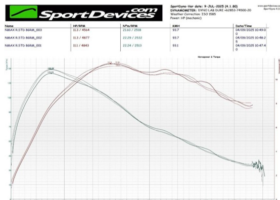
Gambar 2. Grafik Rata-rata Torsi dan Daya 8g Uji 01-03
