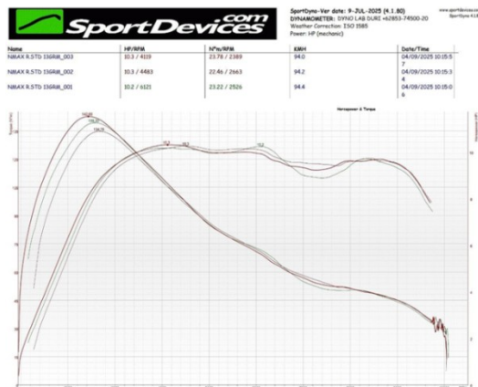
Gambar 3. Grafik Rata-rata Torsi dan Daya 13g Uji 01-03
