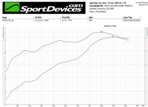
Gambar 2. Grafik Torsi dan Daya Standar
