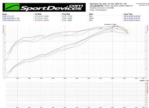
Gambar 5. Grafik Perbandingan Torsi dan Daya
