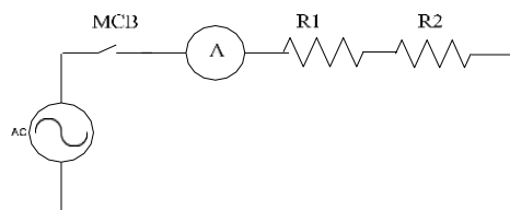
Gambar 7. Pengukuran Arus AC dengan Menggunakan Beban Tunggal
