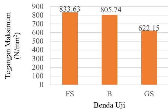
Gambar 4 Diagram rata-rata nilai tegangan maksimum
