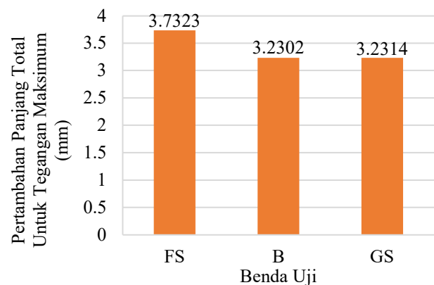
Gambar 6 Diagram nilai pertambahan panjang total tegangan maksimum.
